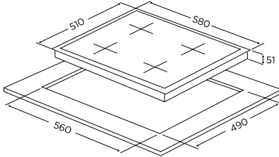
60 cm VITRO SERAMİK OCAK
