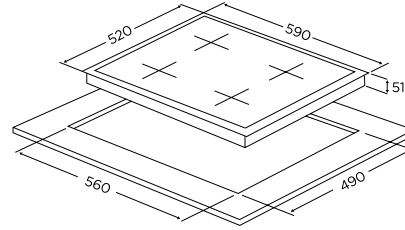
60 cm INOX OCAK
