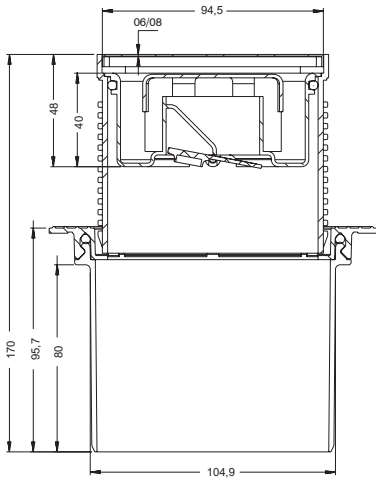
Ø 100 ALT ÇIKIŞ
